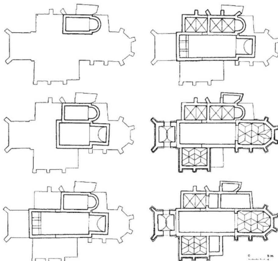
Zalasántó, r.k. templom. A középkori periódusok alaprajzai (Koppány 2003, 29.)
