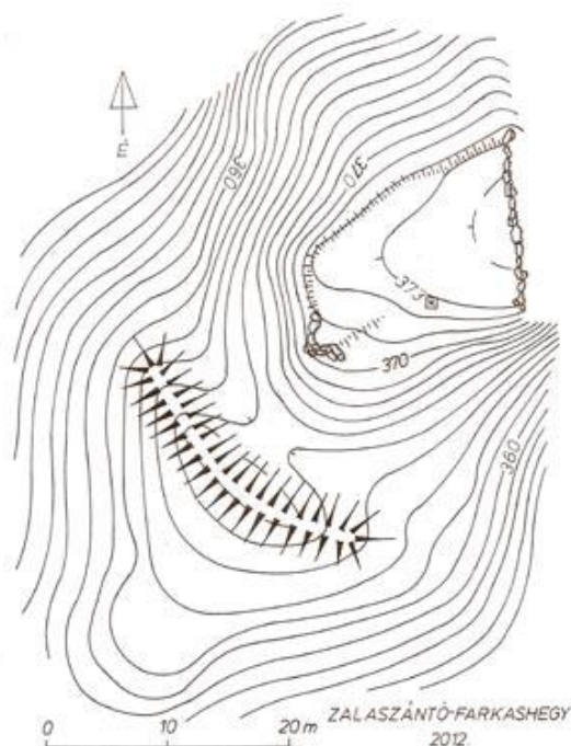
Asszonyvár felmérési rajza
